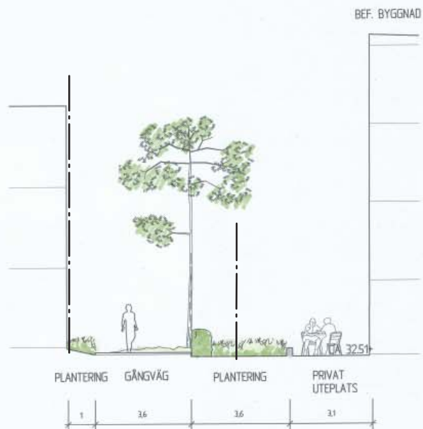
Sektion A-A Skala 1:100 (A1)
