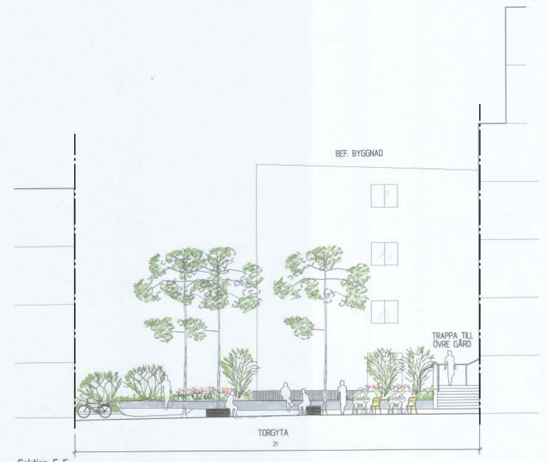
Sektion E-E Skala 1:100 (A1)
