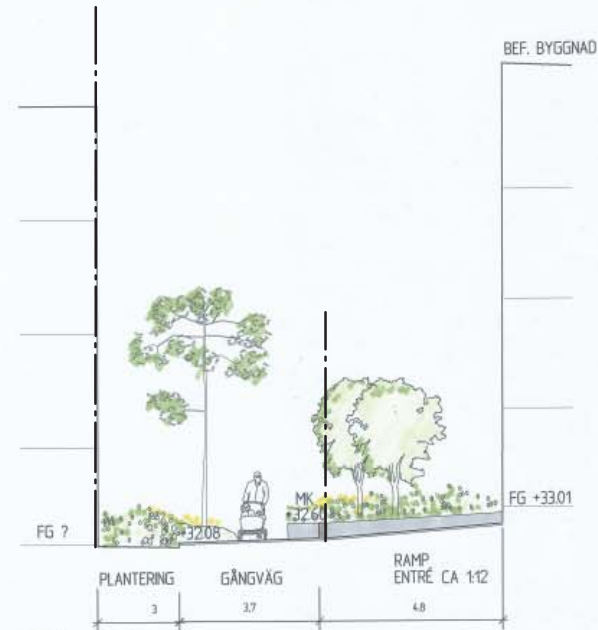
Sektion C-C Skala 1:100 (A1)
